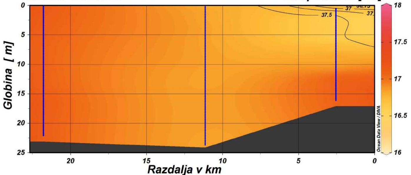
Slanost - izohaline
