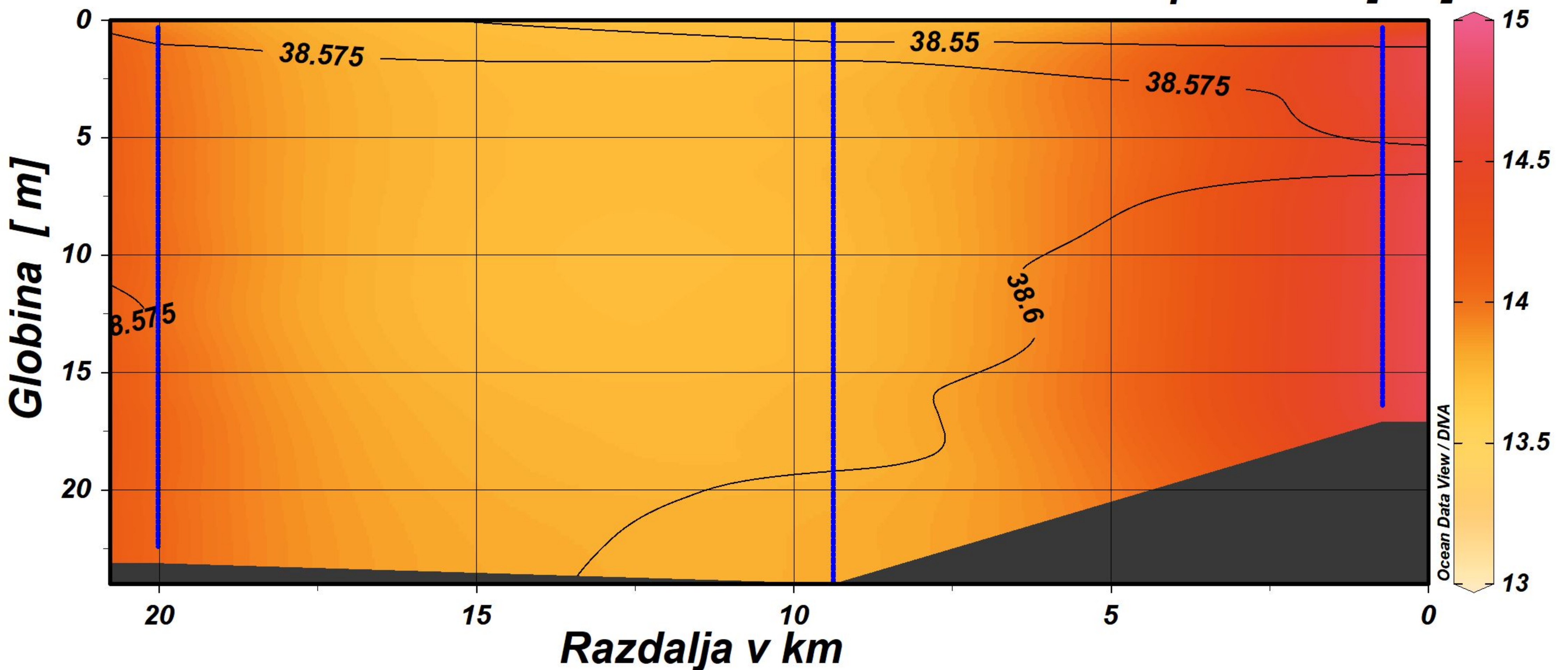
Slanost - izohaline
